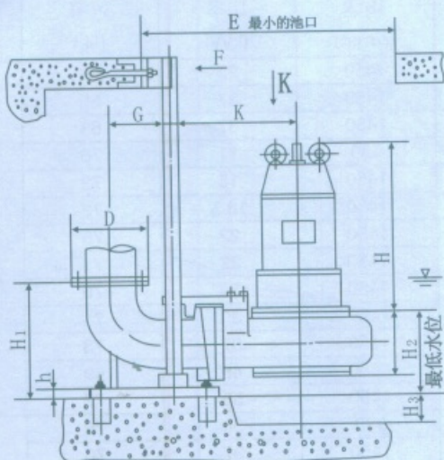
WQ型泵固定式自动安装尺寸表
