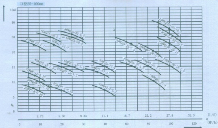
WQ、QW、LW(WL)、YW、GW型泵型谱图
