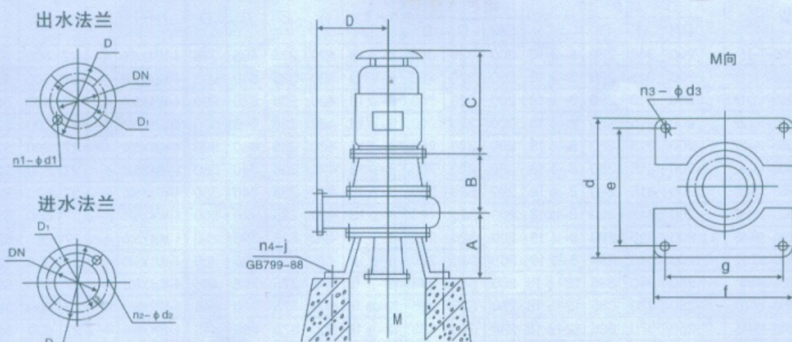
LW(WL)型泵外形及安装尺寸表
