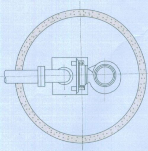
双导轨单泵排水平面图
