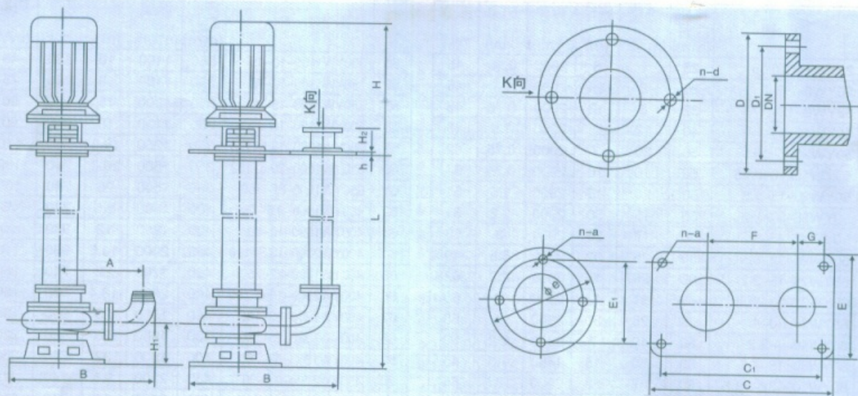
YW型泵外型及安装尺寸表
