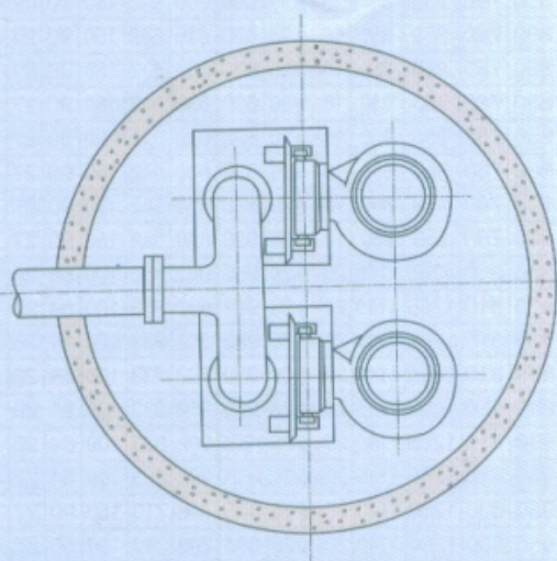
双导轨双泵排水平面图
