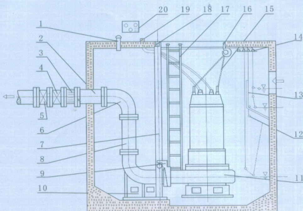
固定式安装示意图
